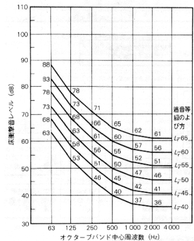
■参考) 床衝撃音遮断性能の周波数特性と等級 (19-2)
