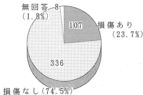
屋内消火栓設備 （設置451対象）
