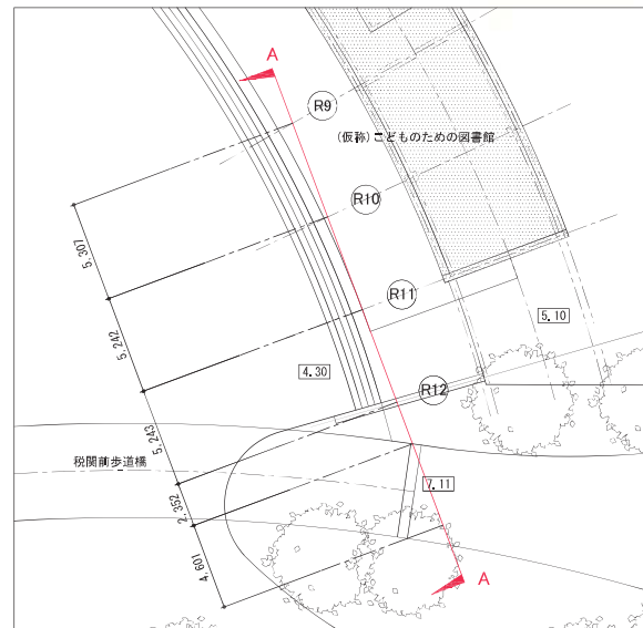
部分平面図 S=1/300
