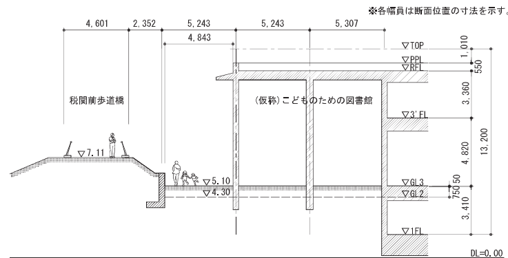
A-A断面図 S=1/250
