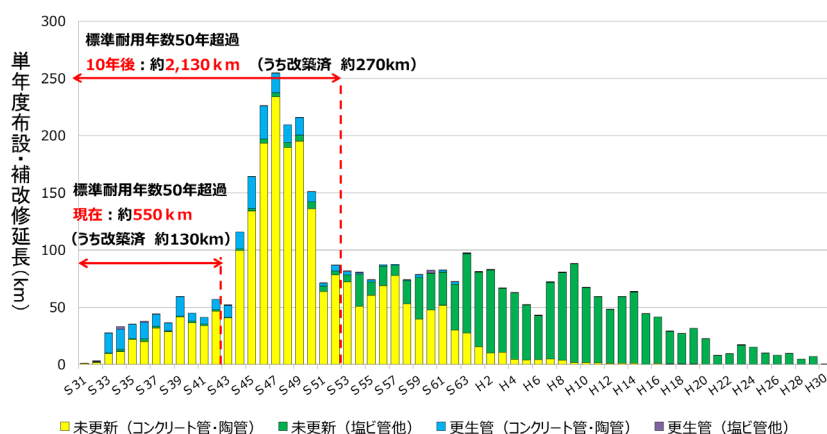
污水管きよの年度別布設状況の推移 (平成 30 年度末時点)
