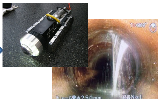
管内のカメラ調査
