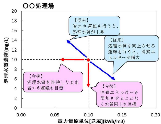
処理水質と消費エネルギーの関係グラフ
