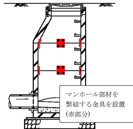
マンホールの耐震補強例
