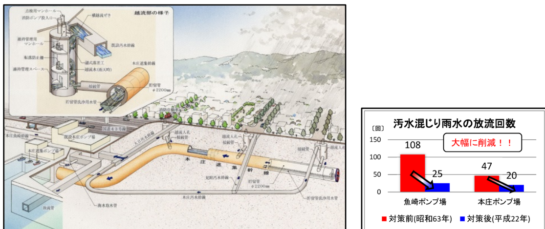
合流式下水道改善事業 (貯留施設の整備) と事業効果
