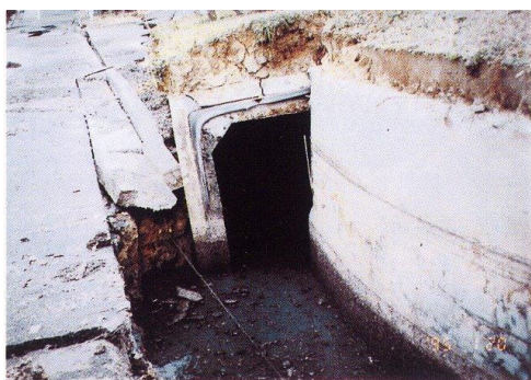
阪神淡路大震災による処理場の被災 (東灘処理場、平成7年1月)
