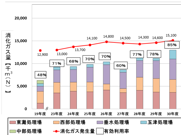
消化ガス発生量と有効利用率の推移
