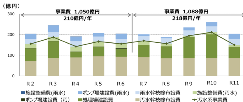
建設改良費の見通し
