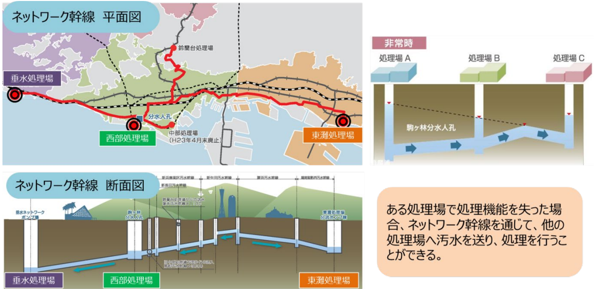
処理場間ネットワークシステムの仕組み
