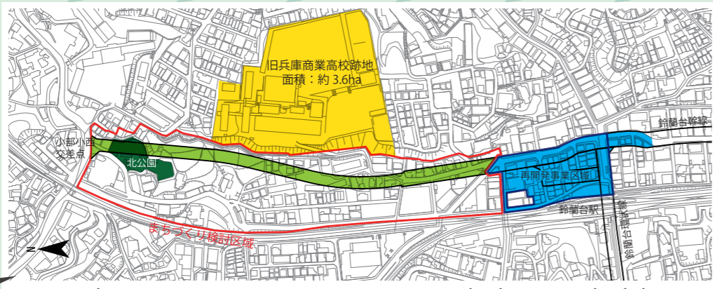
鈴蘭台幹線の計画図
