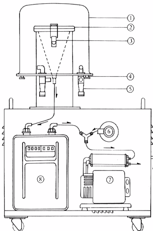
図1 ローボリウムエアサンプラー（新宅FKS型）
