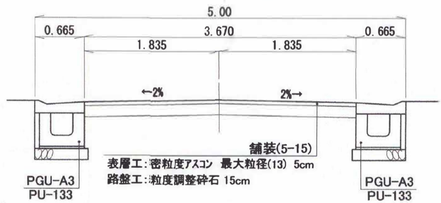
道路横断図 S=1:50
