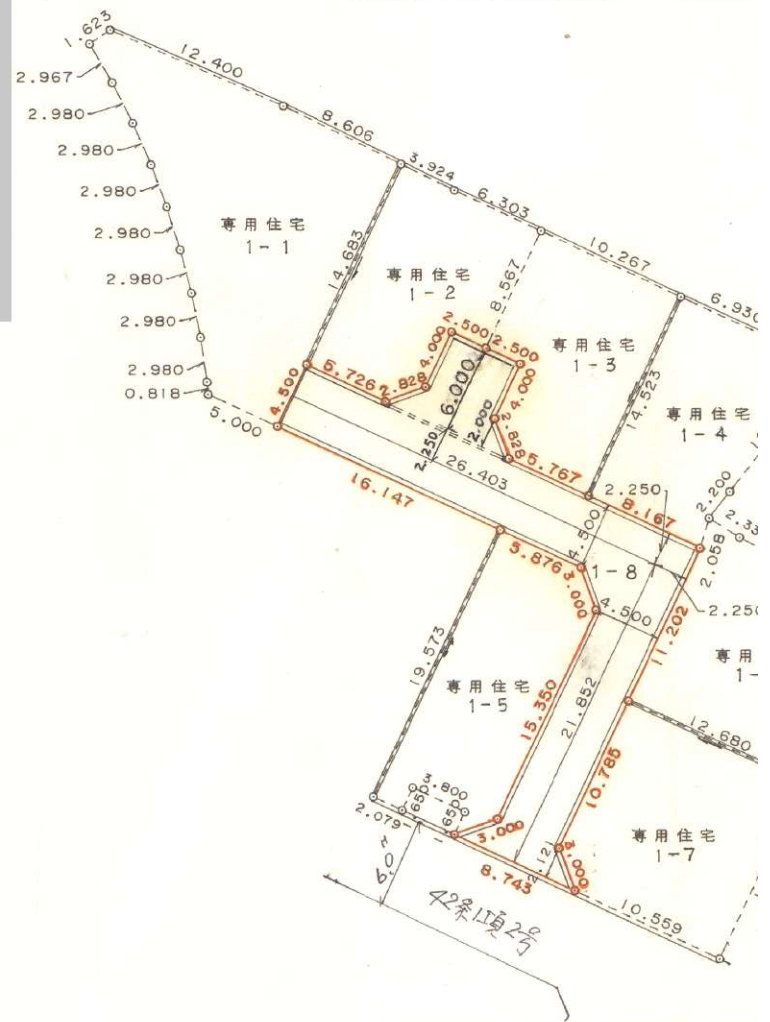
道路平面図 S=1/50
