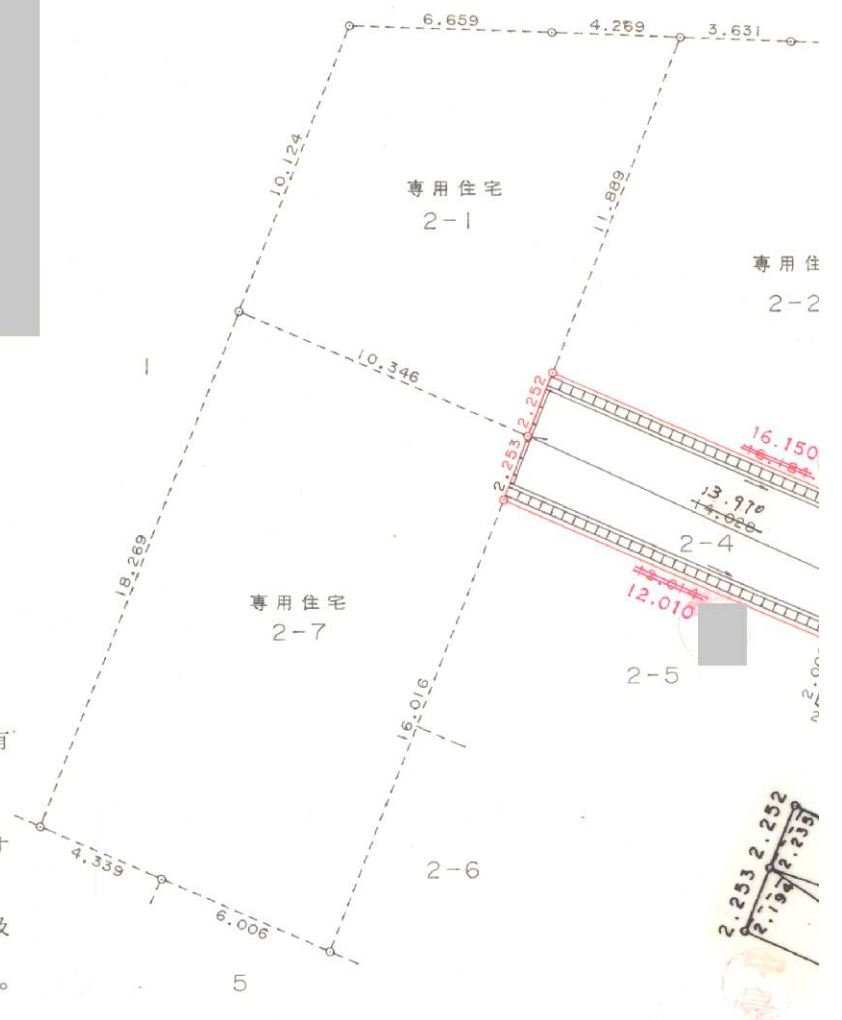
道路平面図 S=1/250
