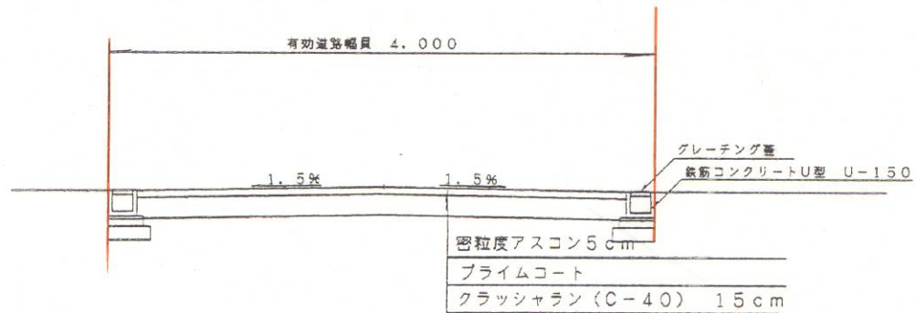
道路3号標準断面図 S=1/30
