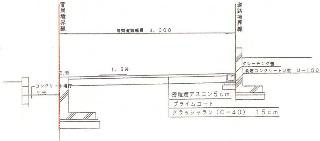
道路B-B'断面図 S=1/30
