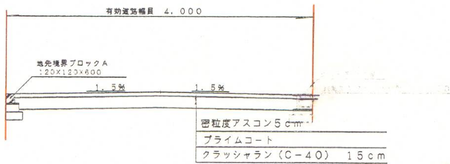
道路3号標準断面図 S=1/30
