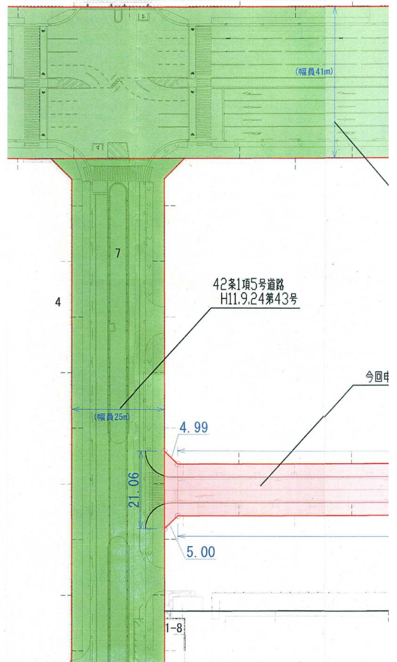
平面図 1/1,000
