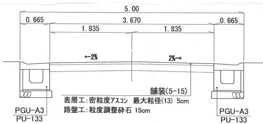
道路横断面図 S=1:50
