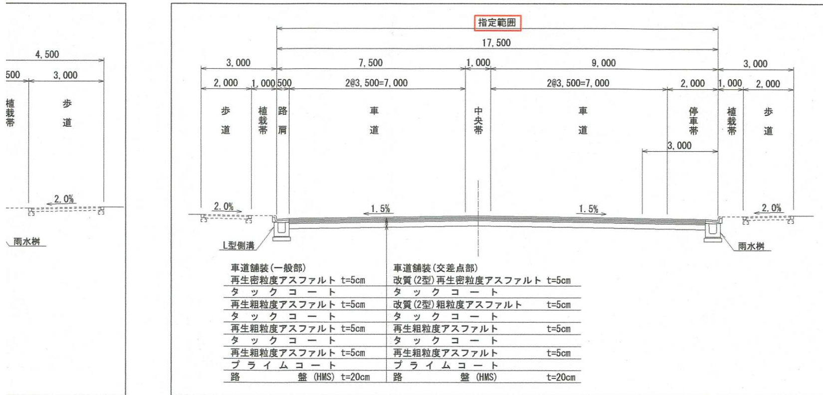
B-B断面
