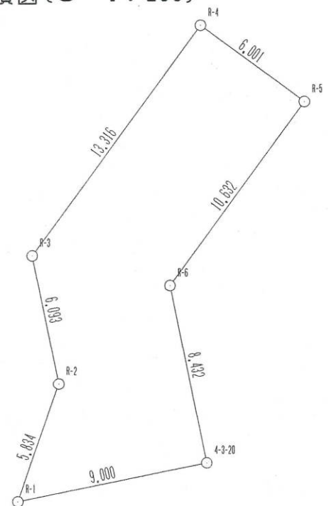
求積図(S = 1 : 250)
