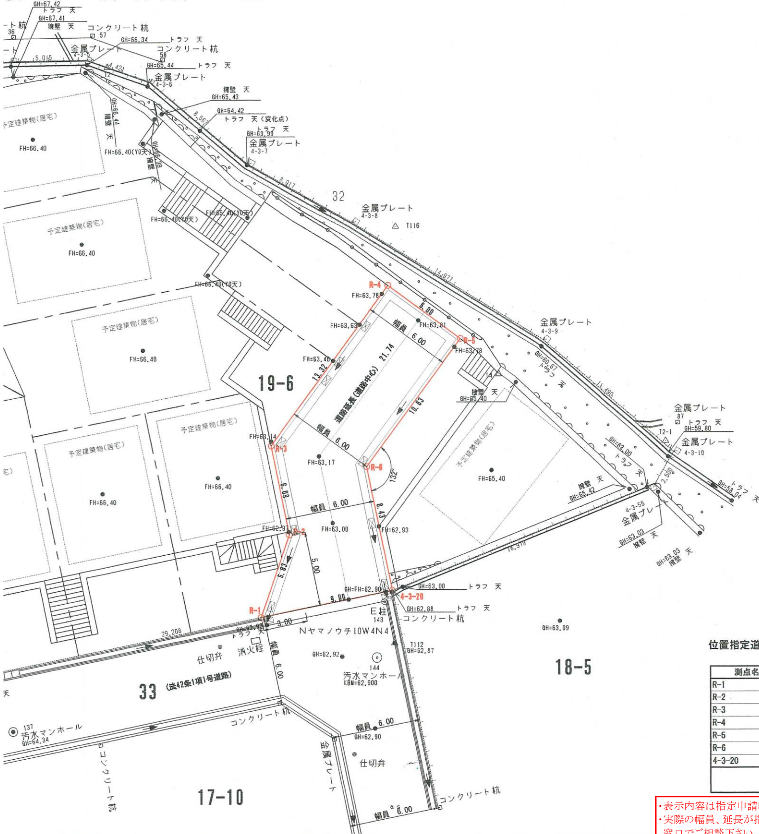
求積図(S = 1 : 250)
