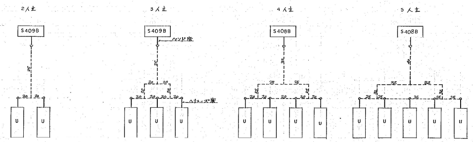
2 小便器洗浄器 図解図 洗浄器は室内埋込み式L管材質はVP-Wとする
